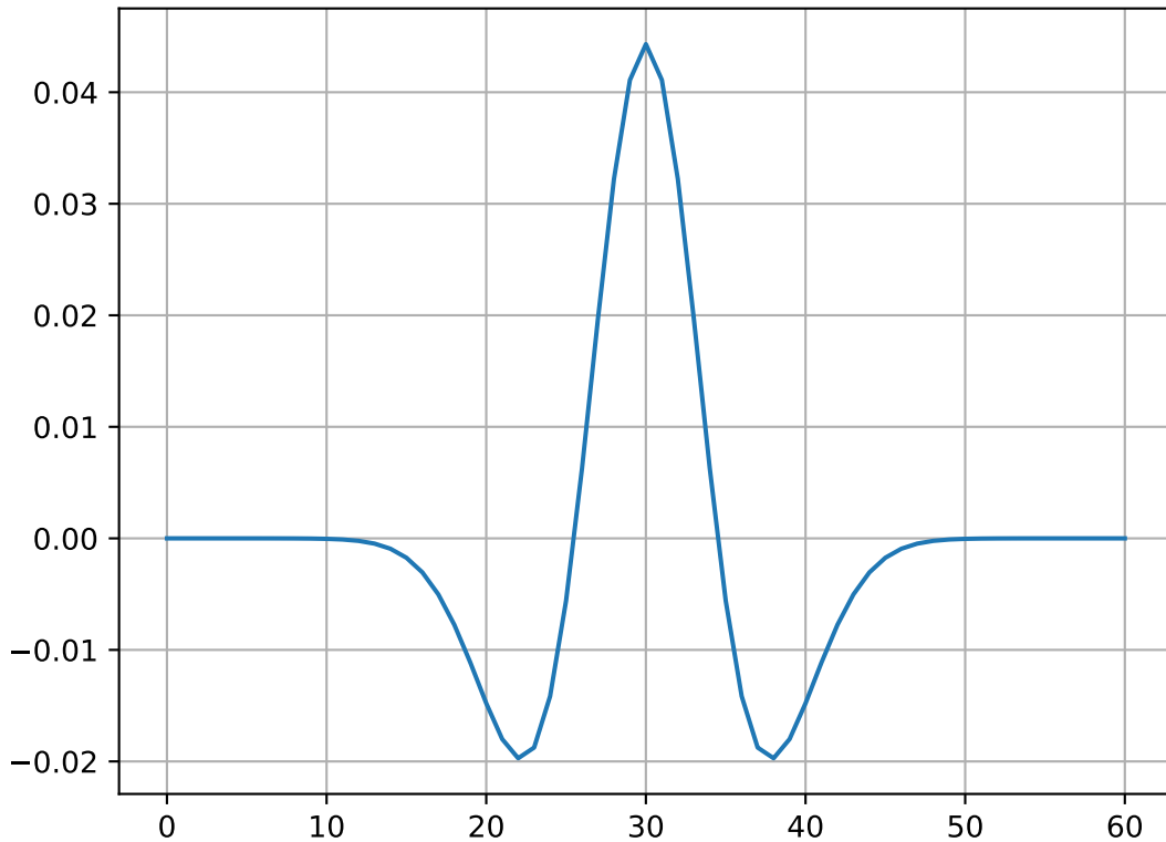
Mexican Hat Wavelet
